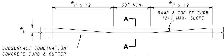
ELEVATION
